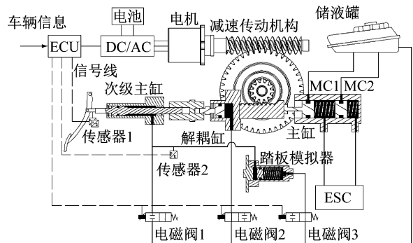
图 2 集成式电子液压制动系统(I-EHB) Fig.2 Integrated-electro-hydraulic brake system (I-EHB)
